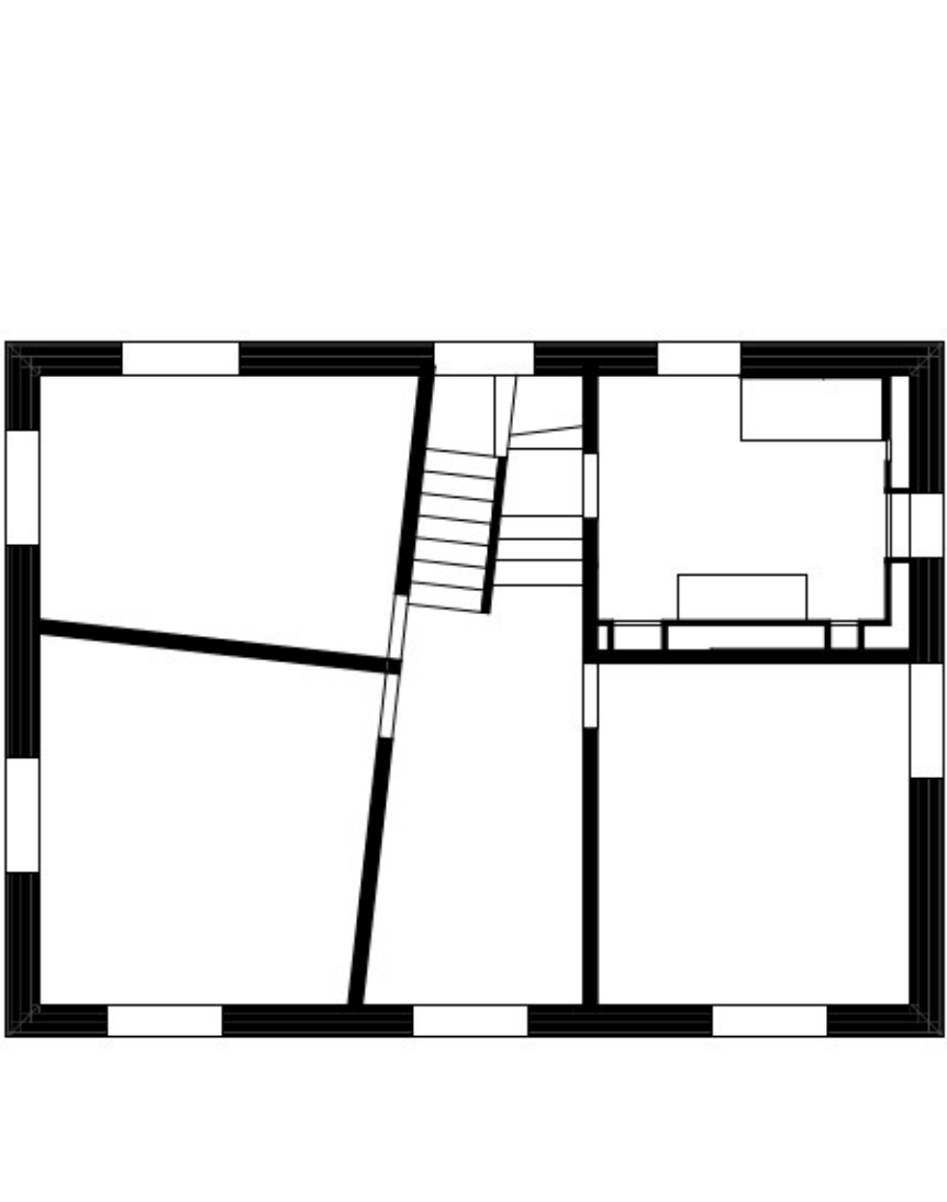
Obergeschoss
