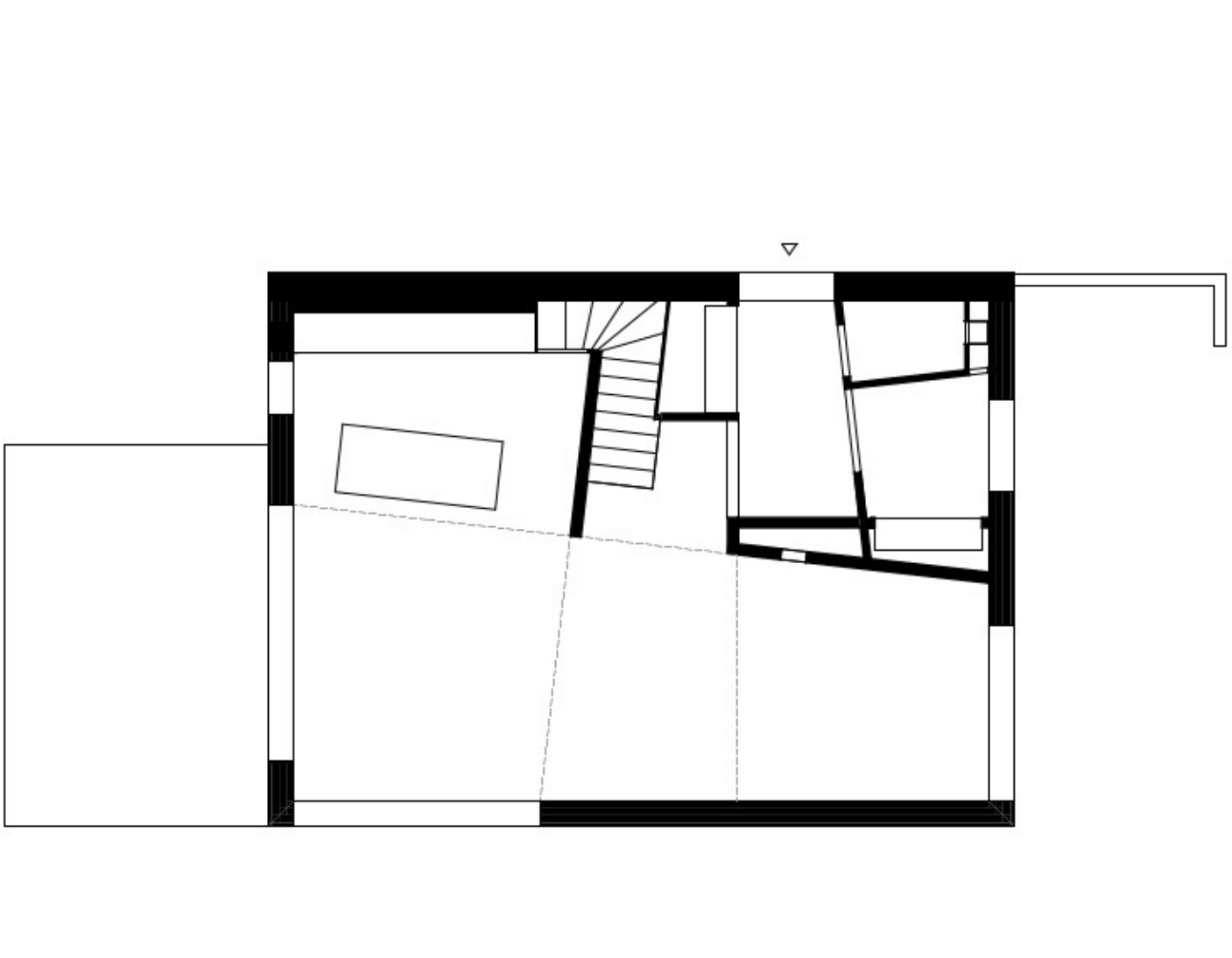
Erdgeschoss
