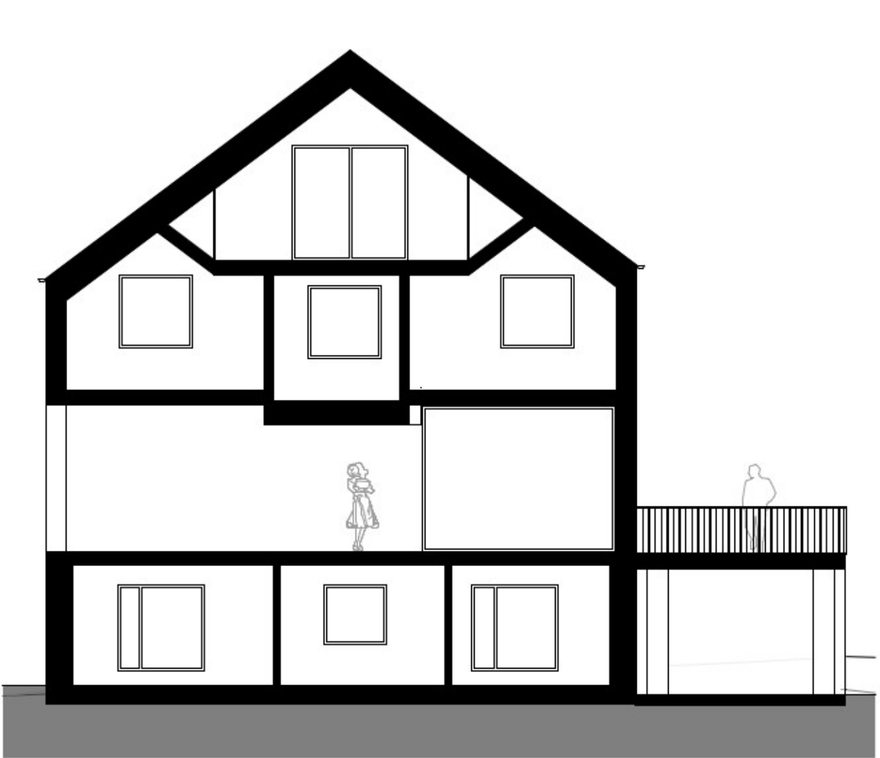
Querschnitt
