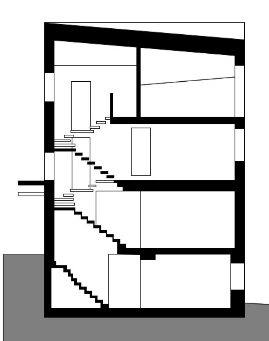
Längsschnitt
