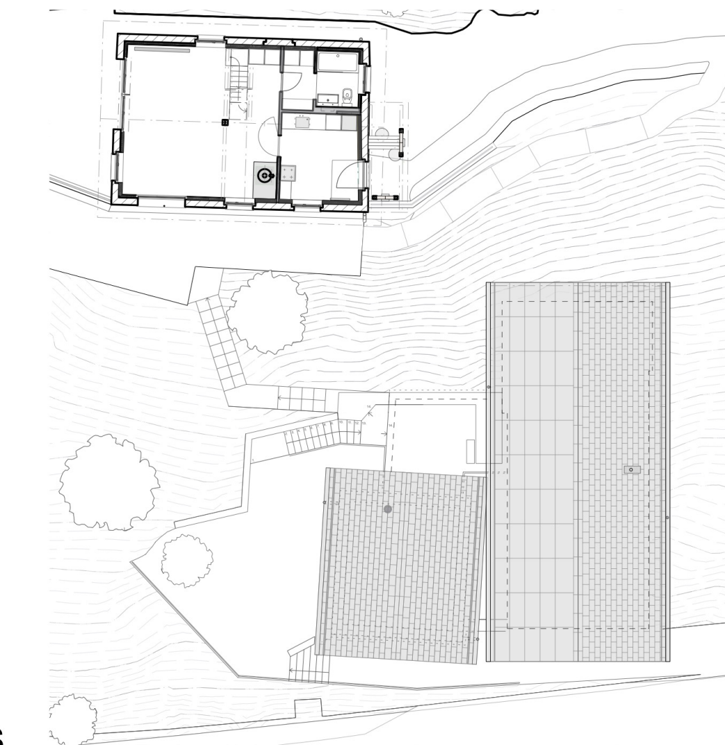
GRUNDRISS DACHAUFSICHT & GÄSTEHAUS
