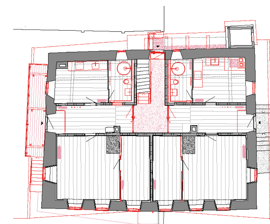
EG - Wohngeschoss mit Nebenkammer - Whg 1, 2
