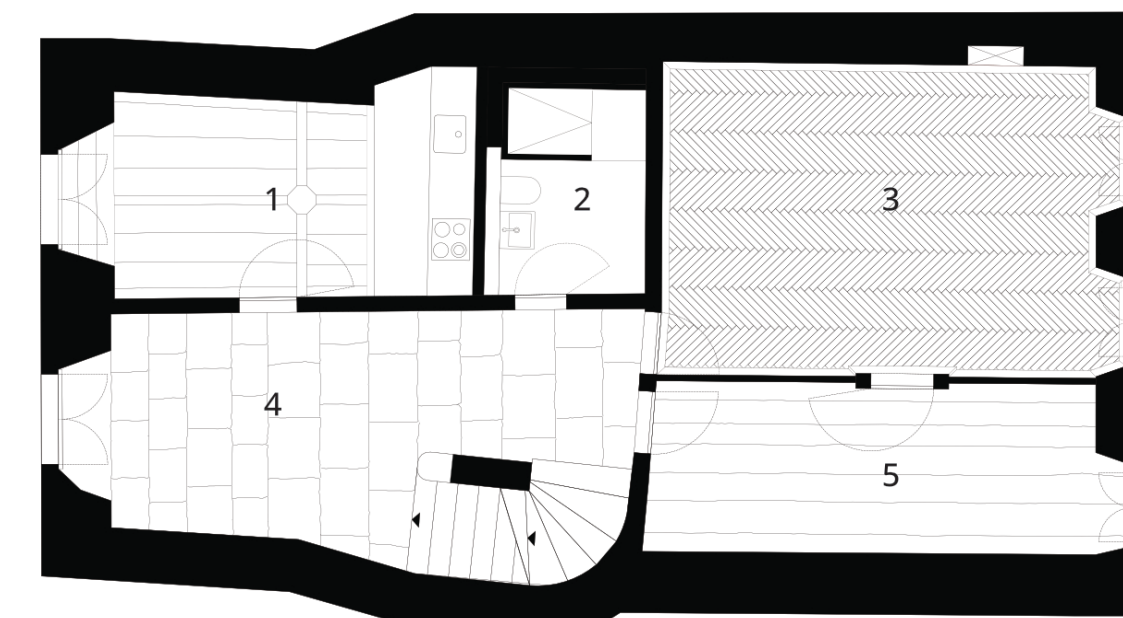
Grundriss 2.OG 1. Küche / Esszimmer 2. Badezimmer 3. Stube 4. Gemeinschaftlicher Flur 5. Nebenstube
