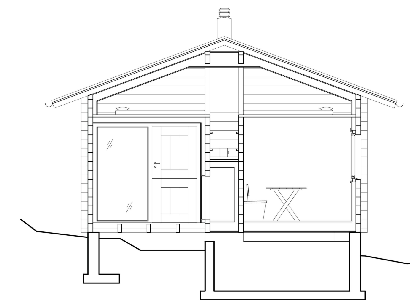
Schnitt A-A
