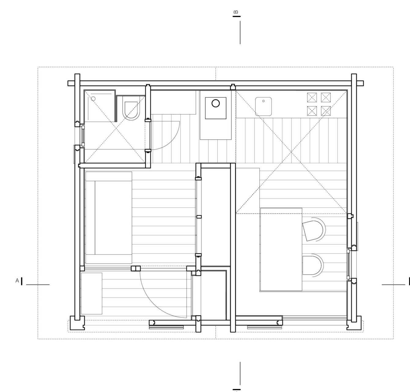
Grundriss Erdgeschoss
