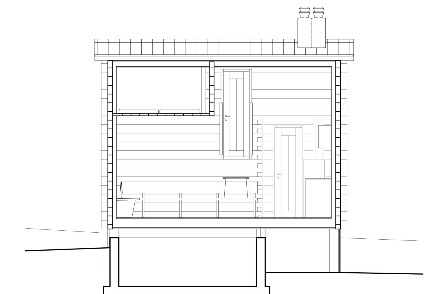
Schnitt B-B 1:50
