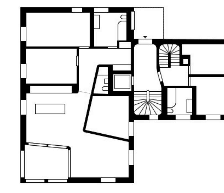
Obergeschoss
