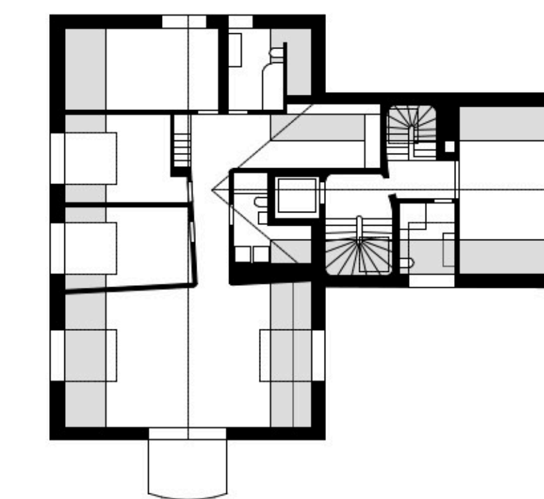
Dachgeschoss
