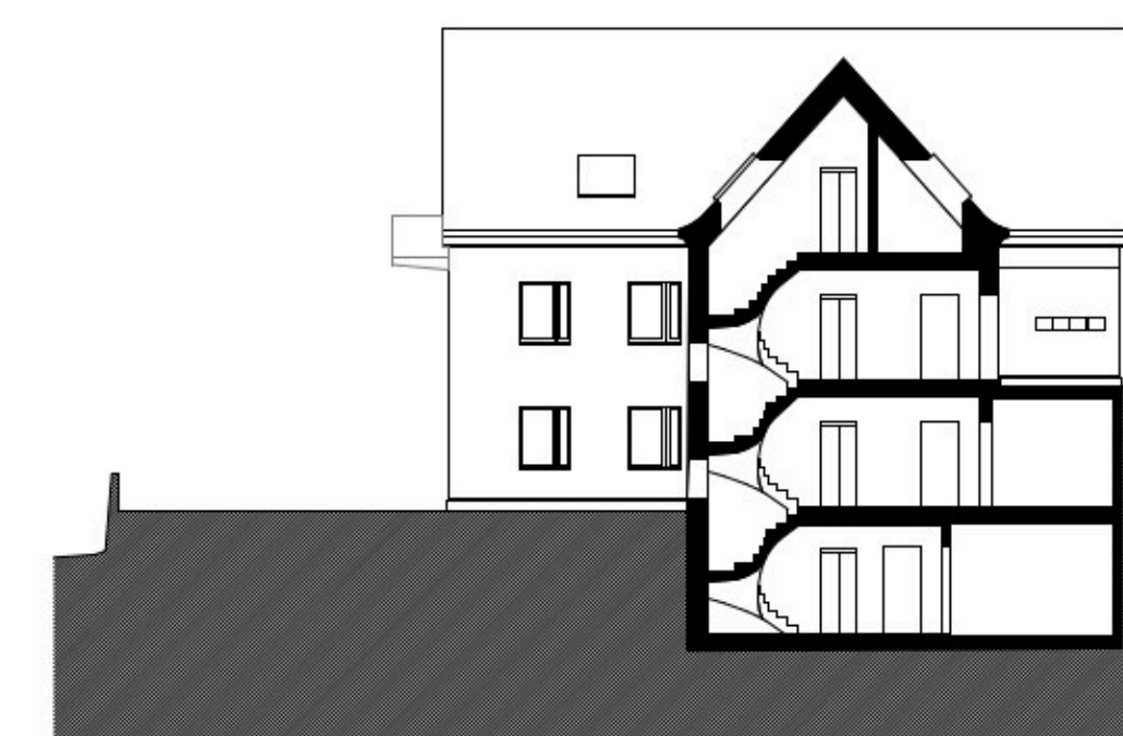
Querschnitt Turmhaus
