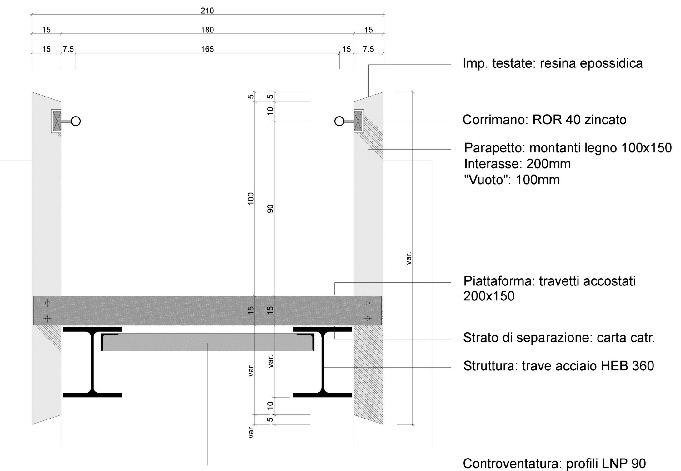
SEZIONE TIPO
