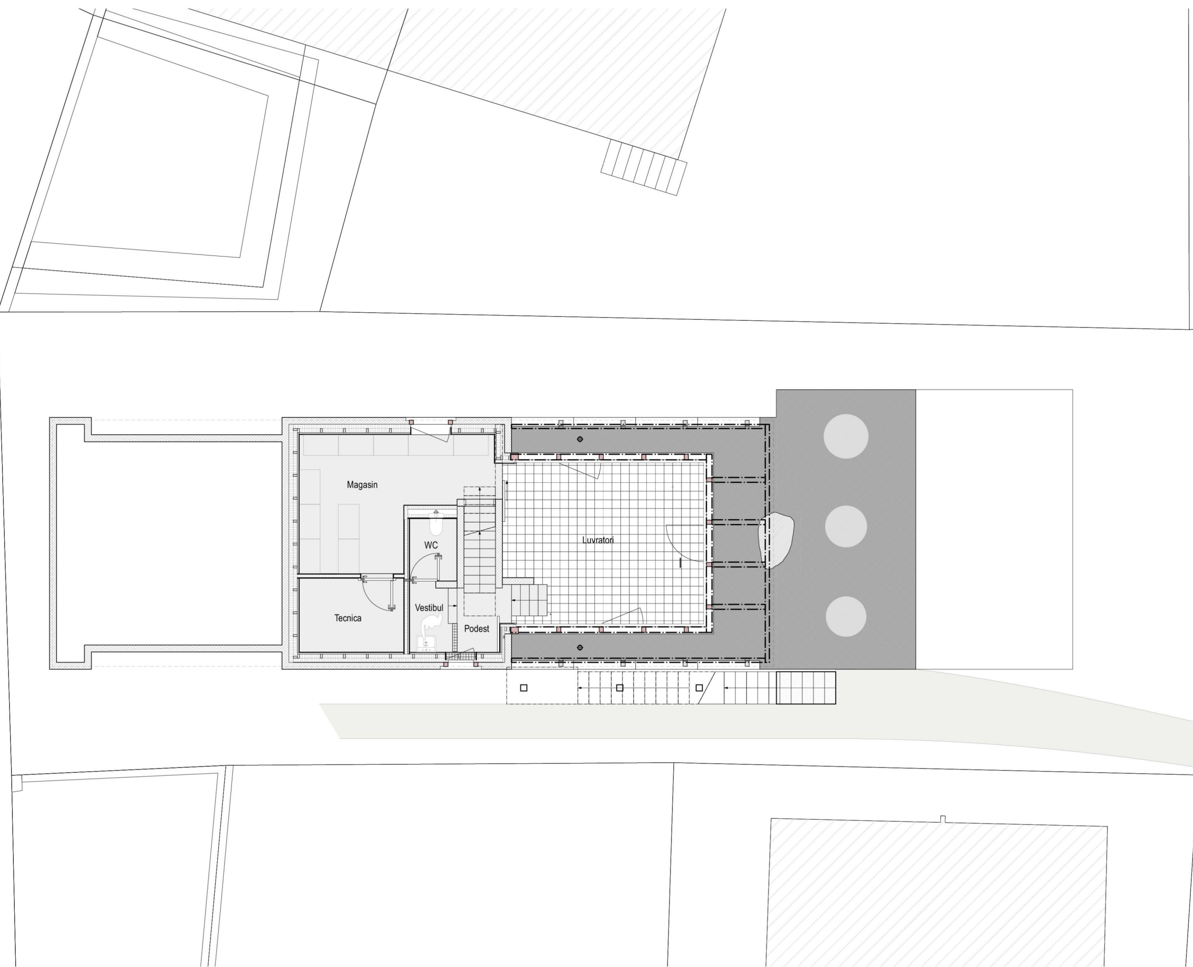
Grundriss Untergeschoss
