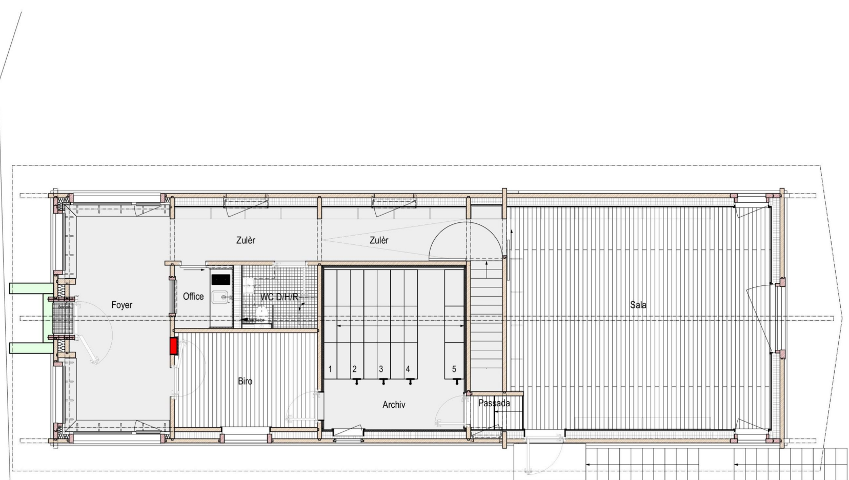
Grundriss Erdgeschoss
