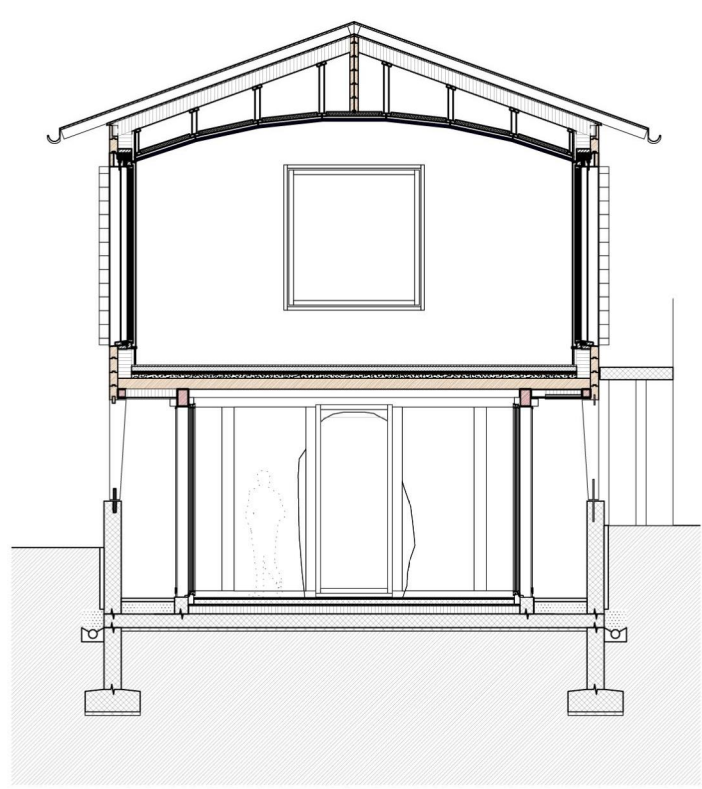
Schnitt durch Saal
