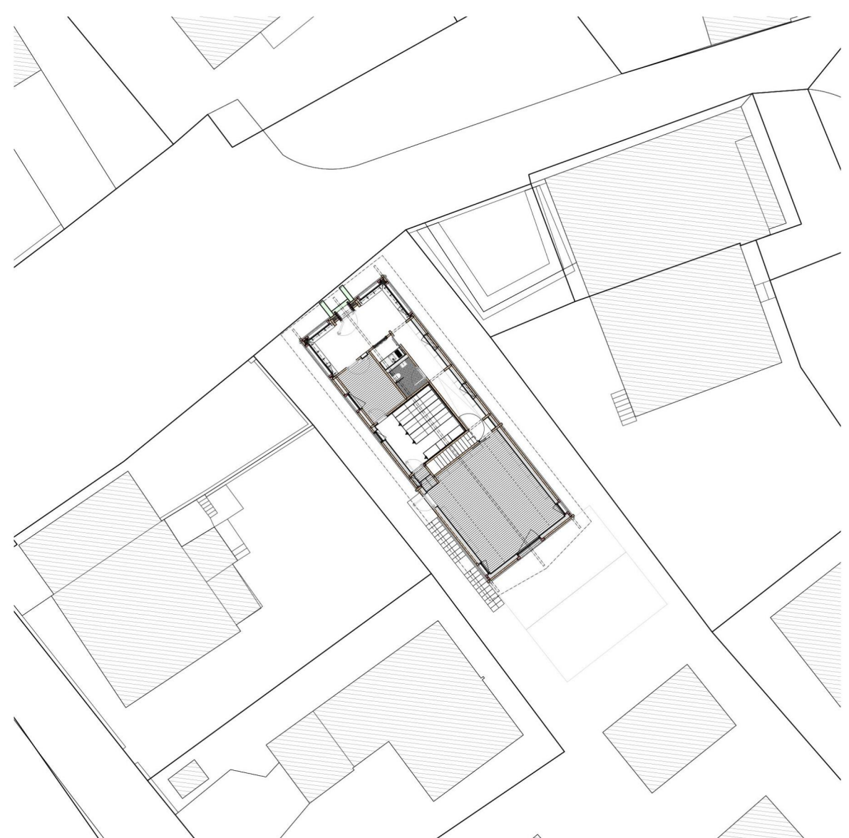
Situation Sedrun, Gemeinde Tujetsch
