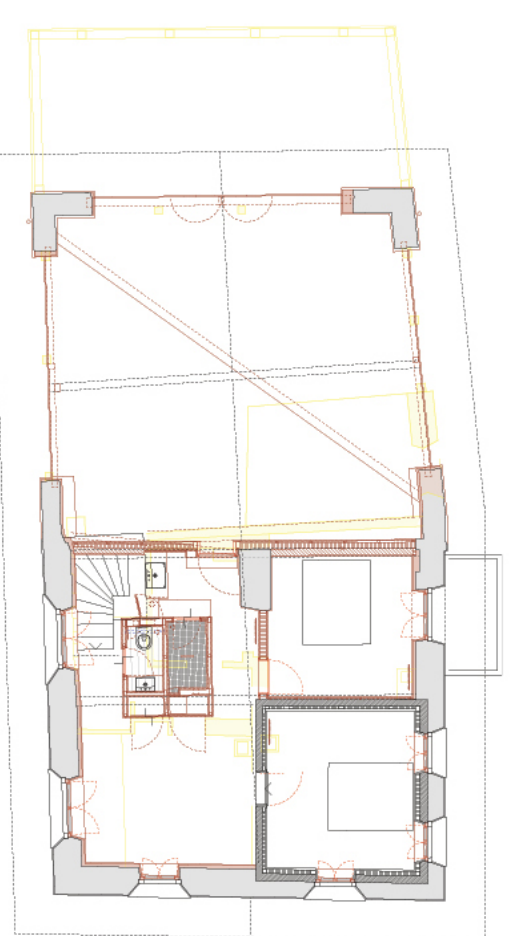
Grundriss Obergeschoss
