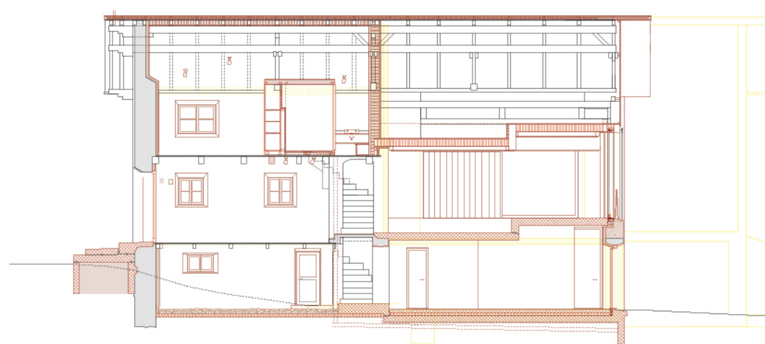
Schnitt Süd - Nord
