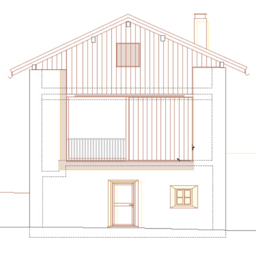
Ansicht Nord
